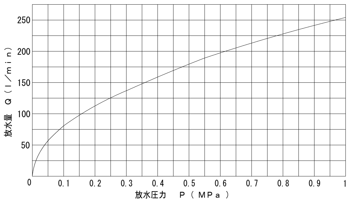
圧力-放水量曲線 流量定数 K=80 ( Q=K\sqrt{10P} )
